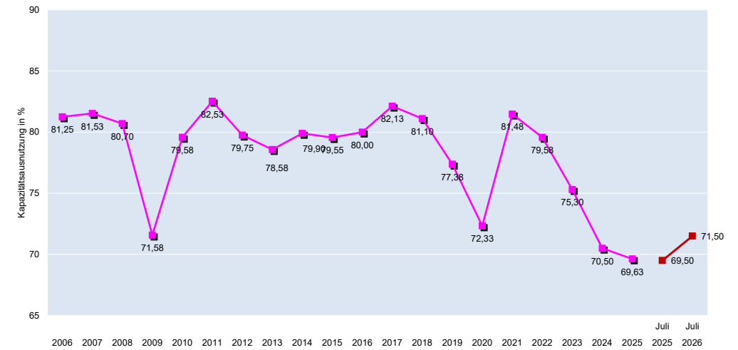
Kapazitätsausnutzung Kunststoffwaren 2006 - 2026
