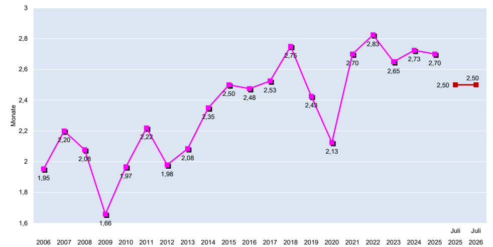
Auftragsbestände Kunststoffwaren 2006 - 2026
