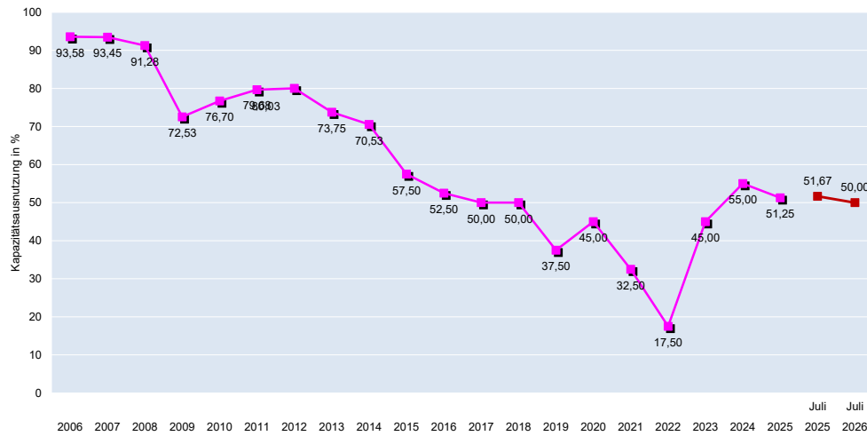
Kapazitätsausnutzung Tapete 2006 - 2026
