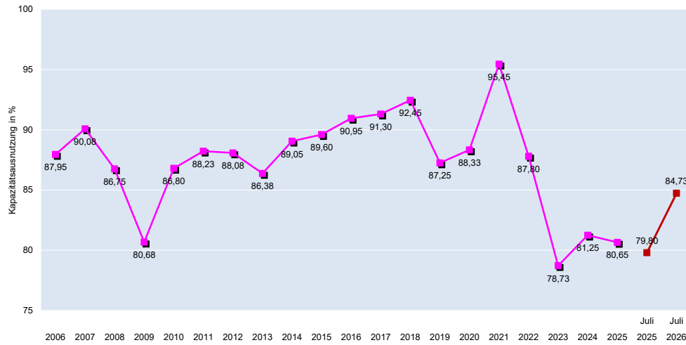
Kapazitätsausnutzung Wellpappe 2006 - 2026
