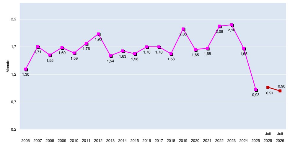
Auftragsbestände Faltschachteln 2006 - 2026
