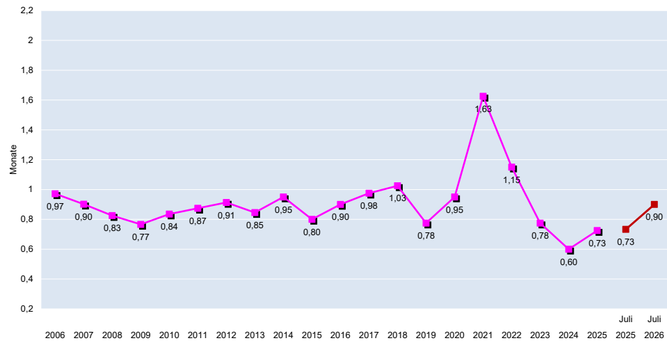
Auftragsbestände Wellpappe 2006 - 2026
