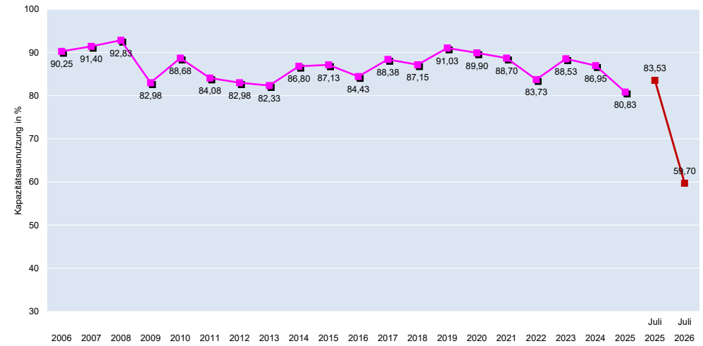
Kapazitätsausnutzung Faltschachteln 2006 - 2026
