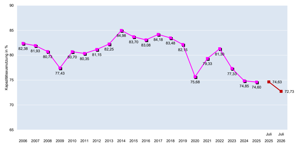
Kapazitätsausnutzung Druckgewerbe 2006 - 2026
