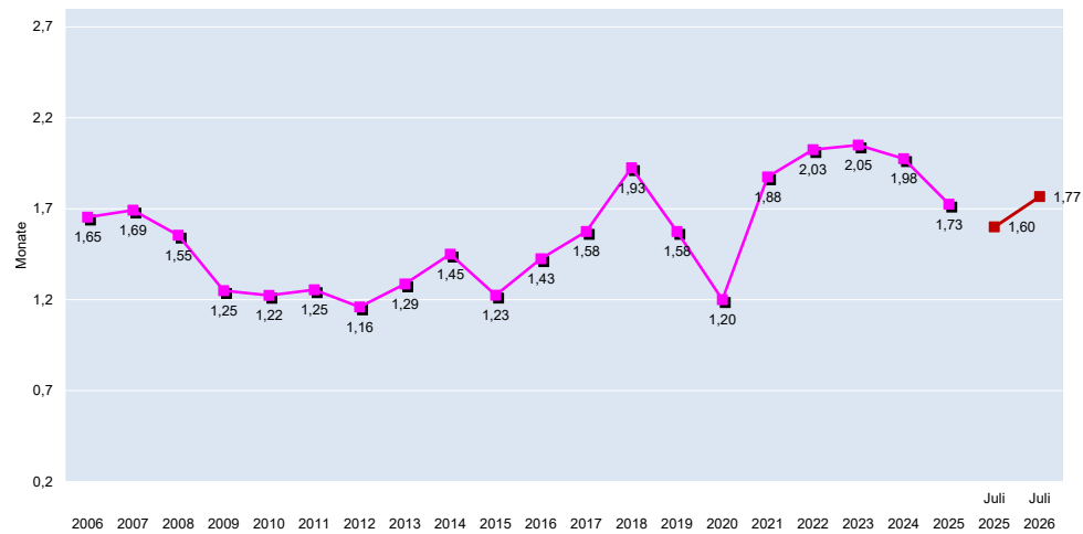
Auftragsbestände Druckgewerbe 2006 - 2026
