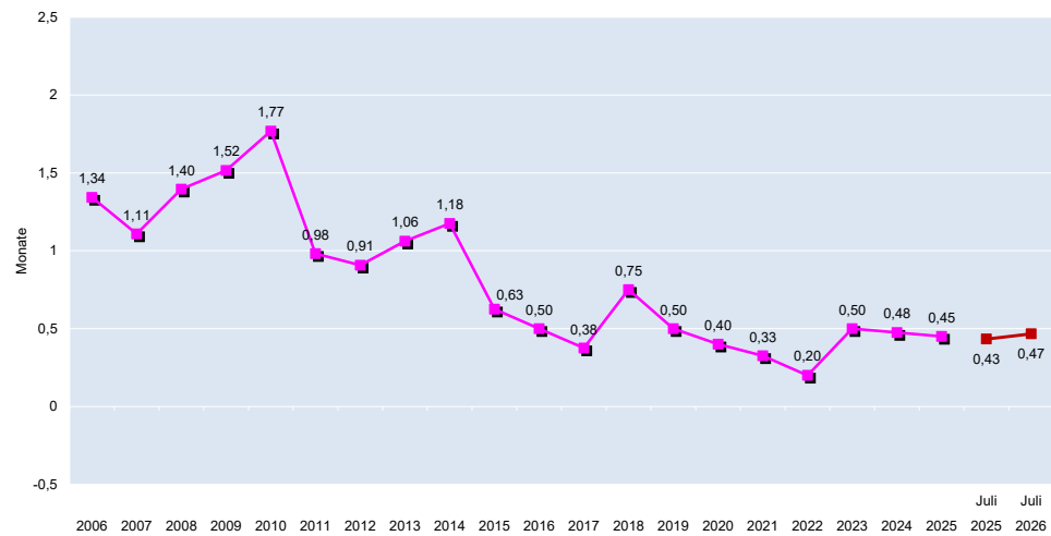
Auftragsbestände Tapete 2006 - 2026
